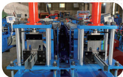
成型后剪 Post Cutter
