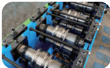
成型主机 Main Roll Forming Mill
